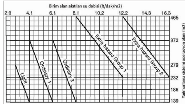
Şekil 12. Birim Alana Akıtılan Su Debisi/Alan Grafiği [8]
