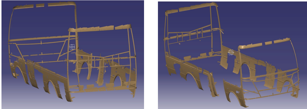
Resim 6: Karkas ve Eteklerin ölçüm sonucu
