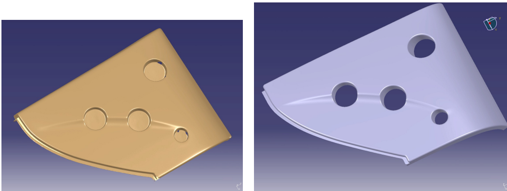
Resim 11: Çamurdan oluşan modelin CAD data ya aktarılması
