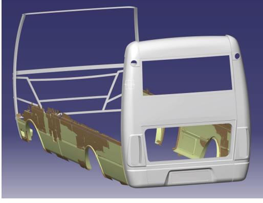
Resim 7 : CAD data oluřturulması
