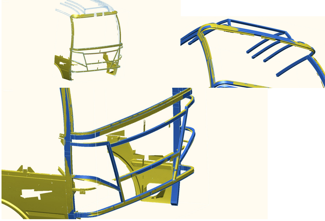
Resim 9: Simetri kontrolu ve Cad data optimizasyonu
