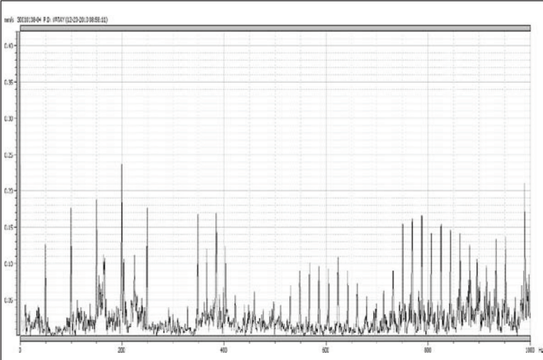
Şekil 4.14. Pompa 3 Dış Yatak Rulman Titreşim Ölçümü Spektrumu (Arızalı Ölçüm)
