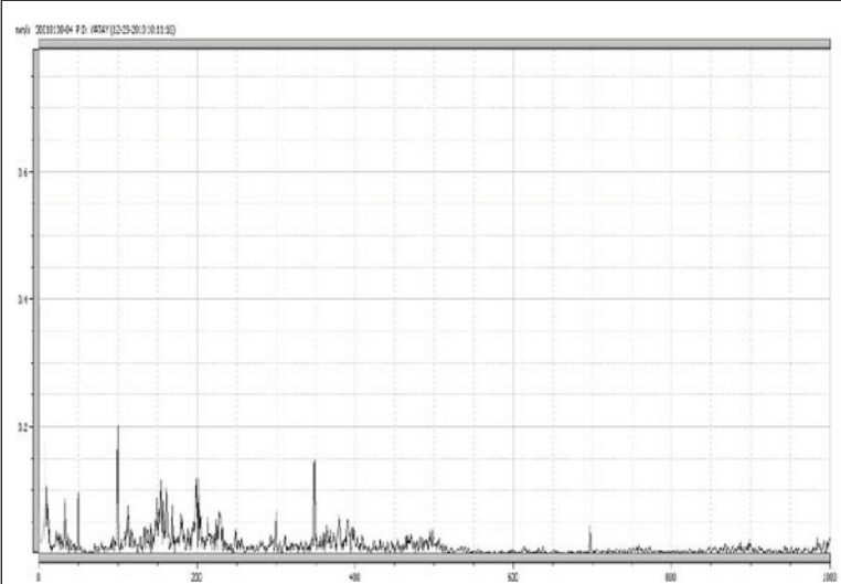
Şekil 4.15. Pompa 3 Dış Yatak Rulman Titreşim Spektrumu (Pompa Değişiminden Sonra)
