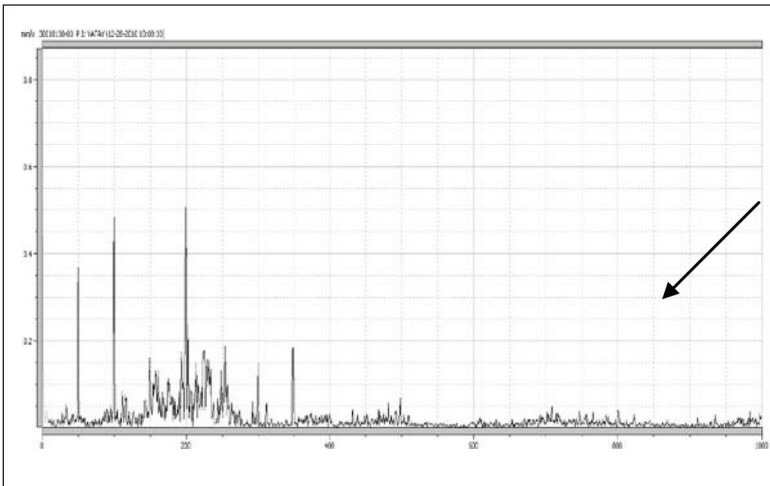
Şekil 4.13. Pompa 3 İç Yatak Rulman Titreşim Spektrumu (Pompa Değişiminden Sonra)
