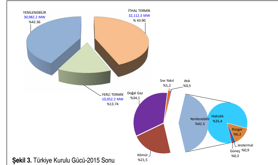
Şekil 3. Türkiye Kurulu Gücü-2015 Sonu
