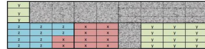
Şekil 6. Kasa 2 İçin Yakınlık Esasına Dayalı Ürün Yerleştirme Modeline Göre Ürün Yerleşimi
