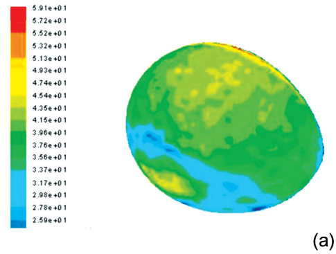
Şekil 3. (a) Soğutma Sırasında ( T=20 dk) Yumurta Yüzeyi Isı Transfer Katsayısı Dağılımı
