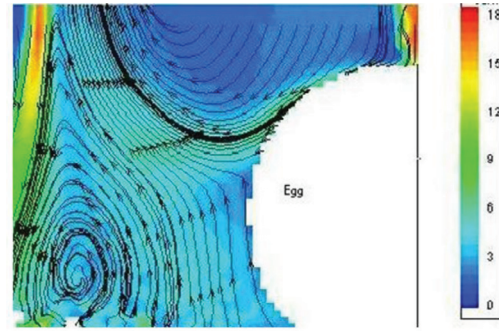
Şekil 2. Yumurta Etrafında Oluşan Akış Profili (19 Numaralı Referanstan Uyarlanmıştır)
