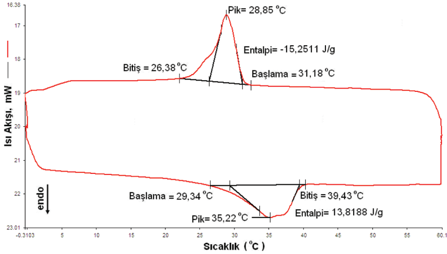
Şekil 3. GA ile Katalizör Kullanılmadan Çapraz Bağlanmış PEG 1.000 İçeren Akrilik Elyafa Ait DSC Grafiği [15]
