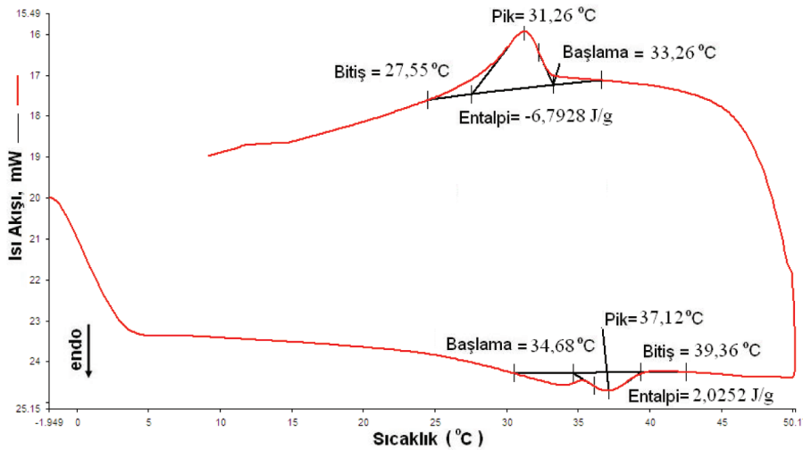
Şekil 4. GA ile Katalizör Kullanılarak Çapraz Bağlanmış PEG 1.000 İçeren Akrilik Elyafa Ait DSC Grafiği [15]
