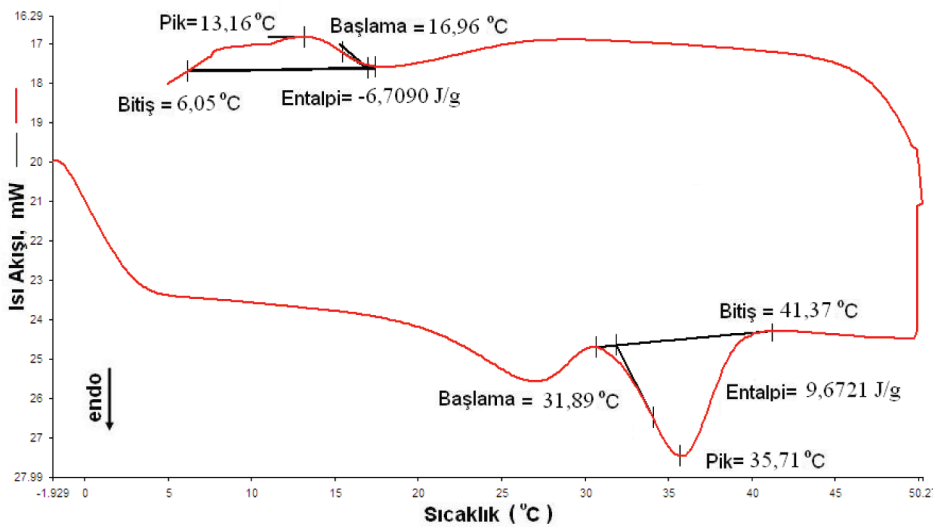
Şekil 2. Arkofix ELF Çapraz Bağlayıcı İle PEG 1.000 Uygulanmış Akrilik Elyafına Ait DSC Grafiği [15]
