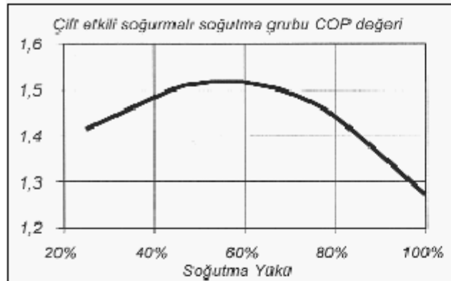
Şekil 2. Çift etkili soğurmalı soğutma gruplarında COP değerinin yüke göre değişimi [3].
