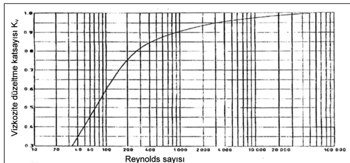
Şekil 3. Viskozite Düzeltme Katsayısı DIN EN ISO 4126-7 Sayfa 29
