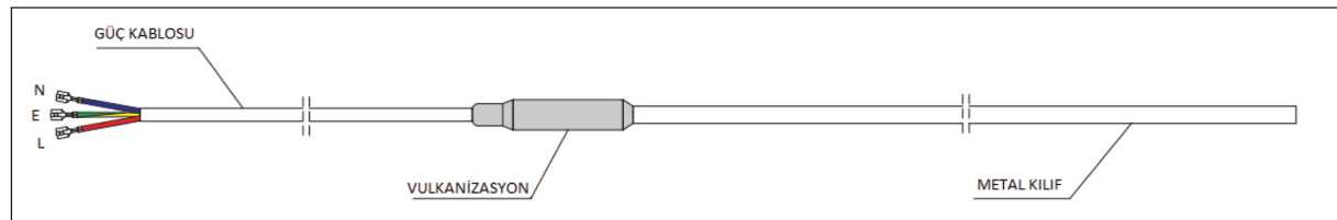
Şekil 1. Defrost Isıtıcı
